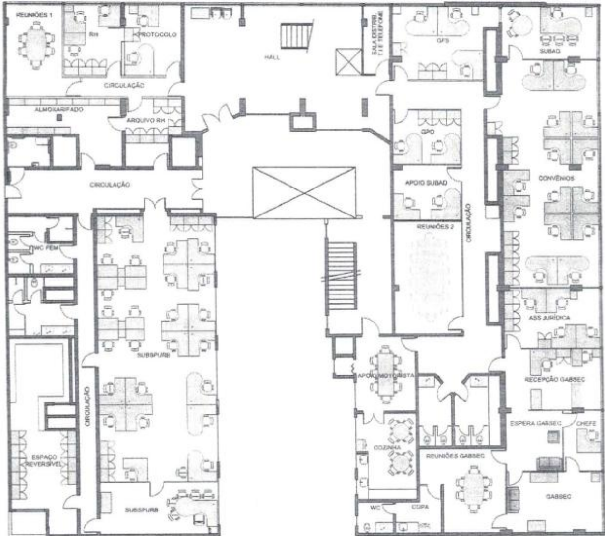
PLANTA BAIXA 20º ANDAR
