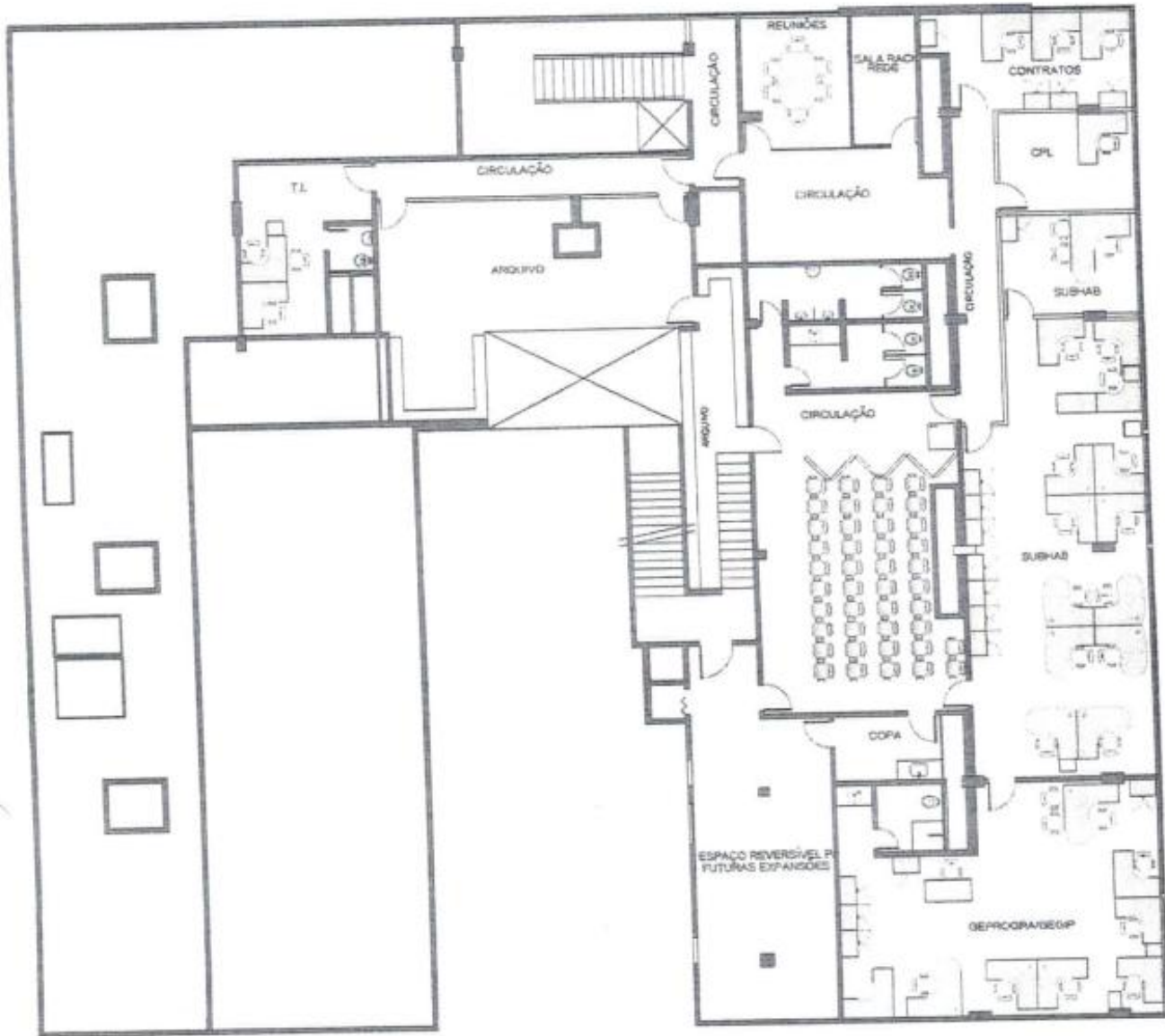
PLANTA BAIXA 21º ANDAR
